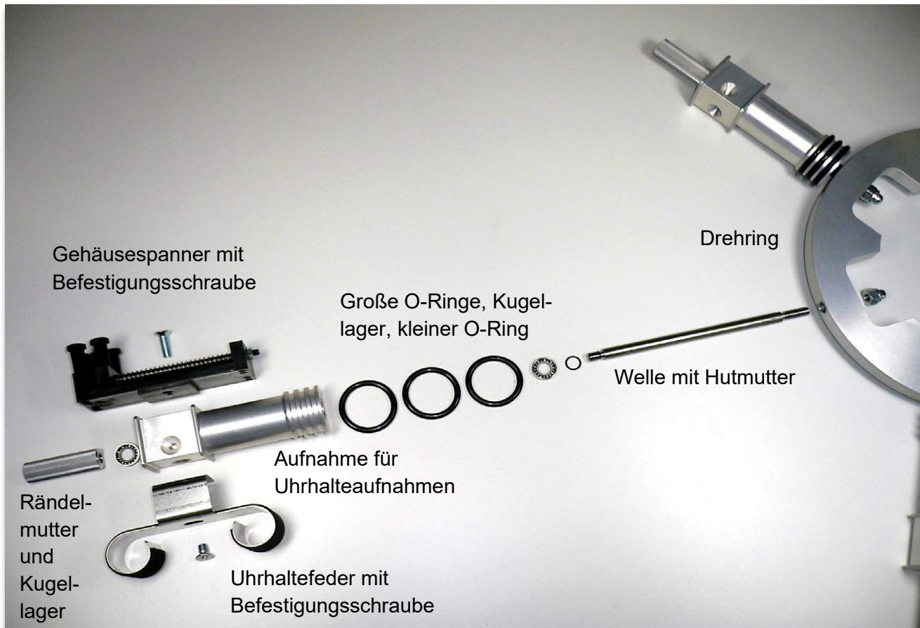
Abb.: Montage eines kompletten Antriebsarmes mit Uhrhaltefedern und/oder Gehäusespanner.
